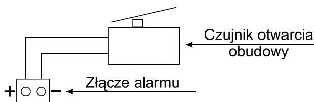
Rys. 4. Złącze alarmu i czujnik otwarcia obudowy – sposób podłączenia
