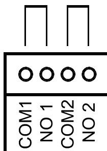
Rys. 6. Schemat połączeń wyjść przekaźnikowych podczas wystereowania przekaźników
