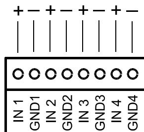
Rys. 5. Schemat połączeń wejść cyfrowych
