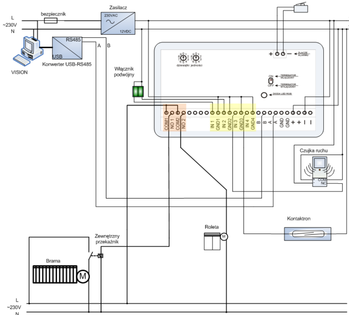
Rys. 10. Schemat aplikacji nr 2
