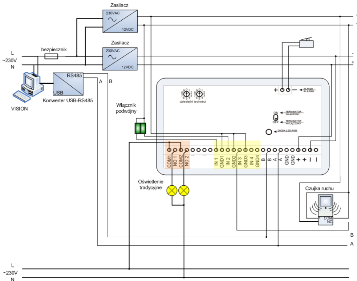
Rys. 9. Schemat aplikacji nr 1
