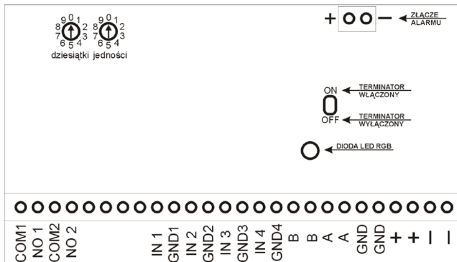
Rys. 1. Widok Neuronu Cyfrowego
