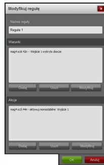
Rysunek 6: Okno konfiguracji reguły Logiki awaryjnej Sterownika Magistrali
